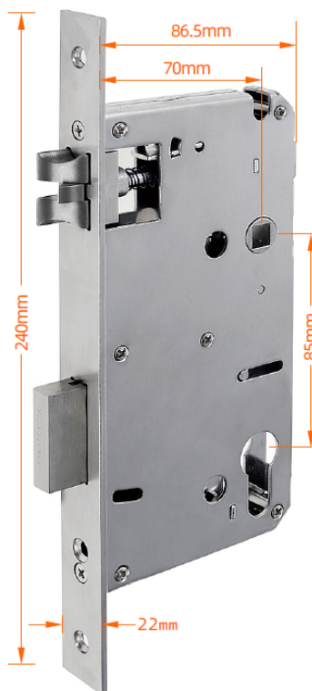
ML-SP-M-70/85-SWING
